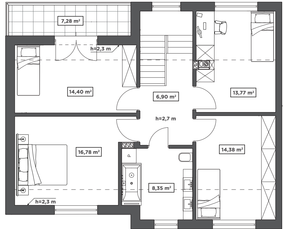
PIĘTRO 1
